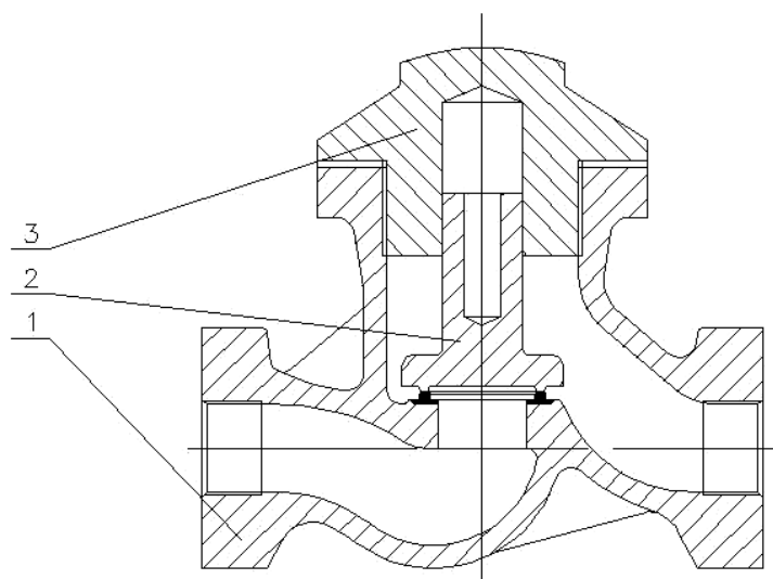
1-阀体 2-阀瓣 3-阀盖
