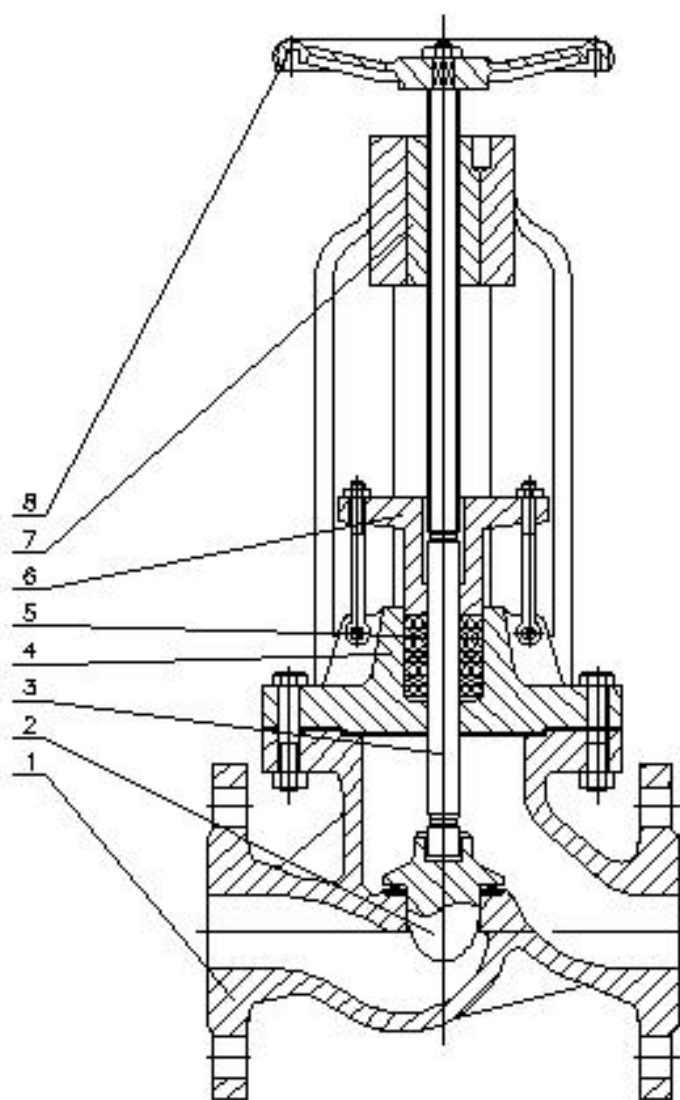
1-阀体 2-阀瓣 3-阀杆 4-阀盖 5-填料 6-填料压盖 7-阀杆螺母 8-手轮
