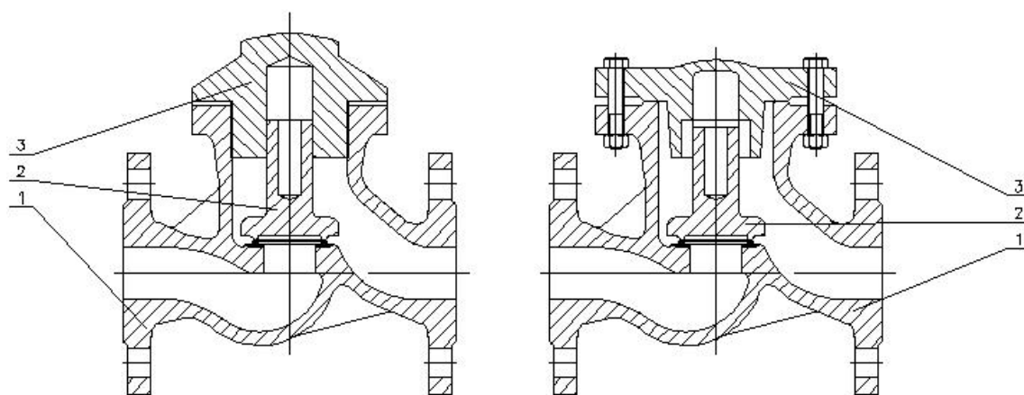
1-阀体 2-阀瓣 3-阀盖
