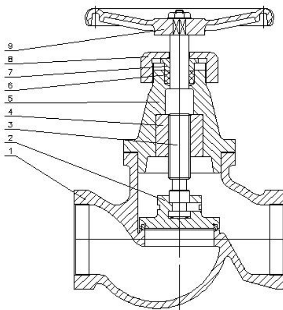
1-阀体 2-阀瓣 3-阀杆 4-阀杆螺母 5-阀盖 6-填料 7-填料压套 8-压套螺母 9-手轮
