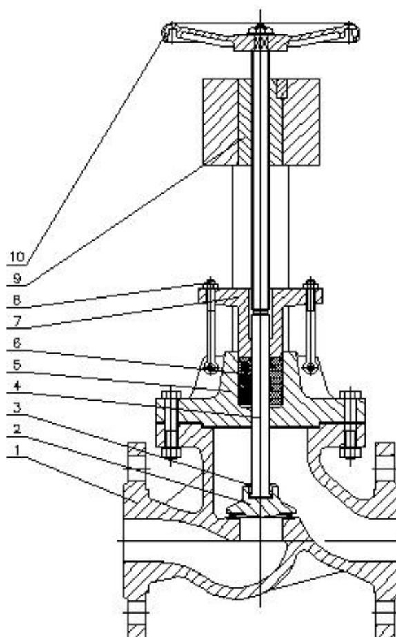
1-阀体 2-阀瓣 3-阀瓣盖 4-阀杆 5-阀盖 6-填料 7-填料压盖 8-活节螺栓 9-阀杆螺母 10-手轮
